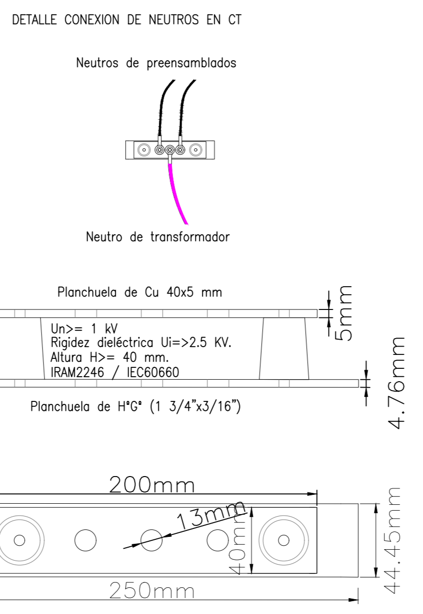
BARRA AISLADA DE NEUTRO
