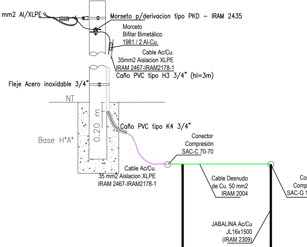
DETALLE PAT EN COLUMNA HFA*
