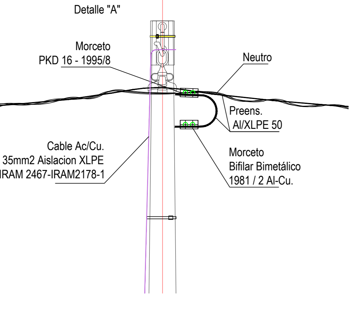
Detalle "A"
