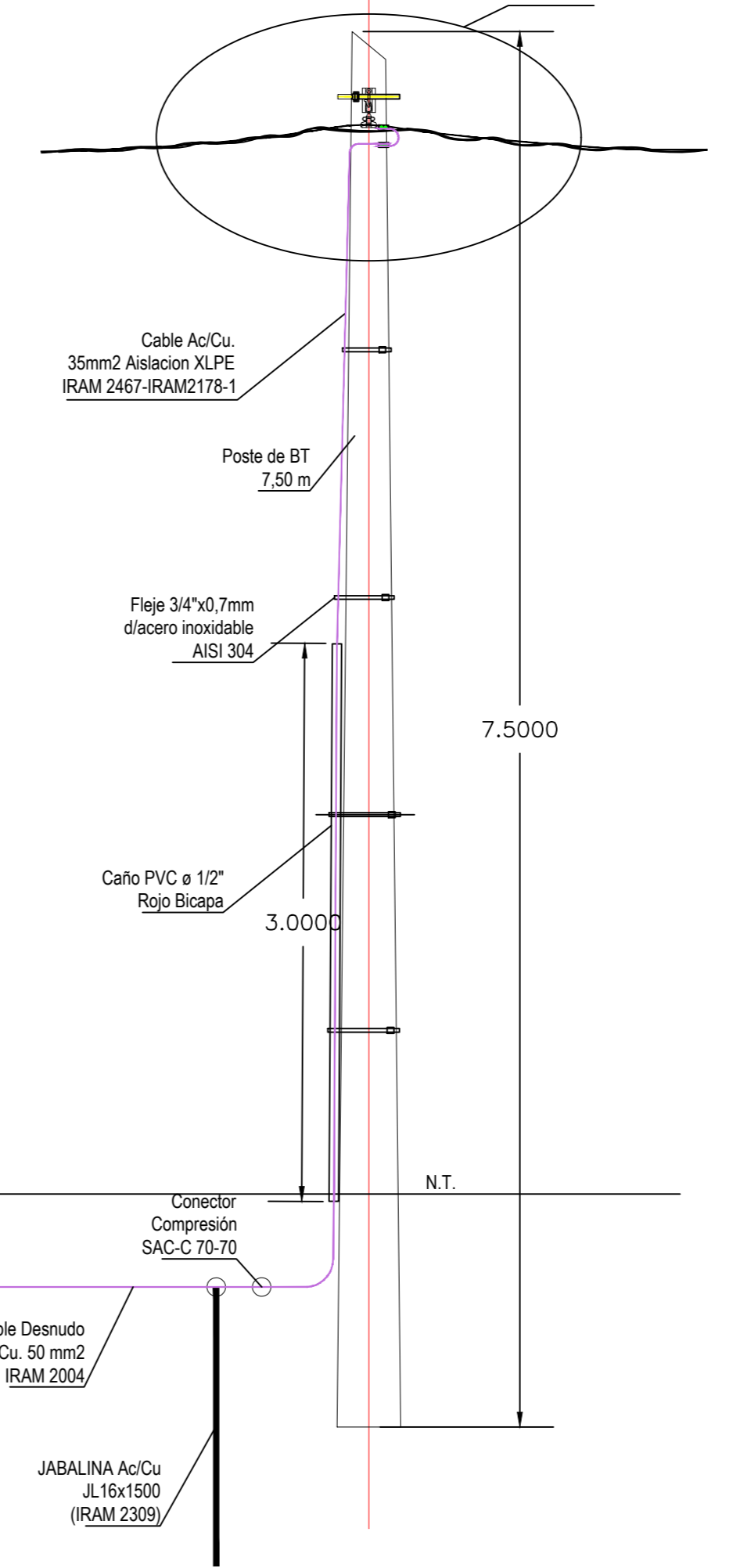
CONJUNTO DE PAT TIPO N-CE
