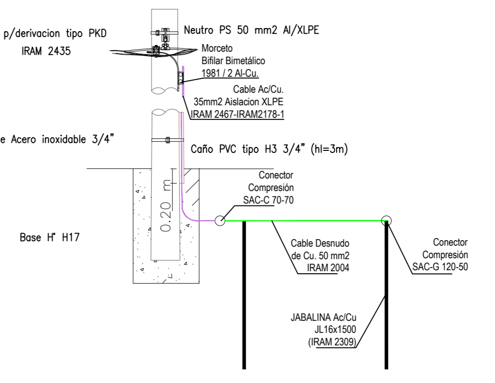
DETALLE PAT NEUTRO EN COLUMNA HFA*
