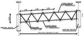
DETALLE VIGA METÁLICA VMR-002-14x75 esc: 1:50
