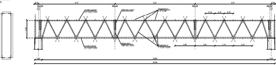
DETALLE VIGA METÁLICA VMR-002-14x75 esc: 1:50
