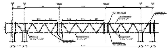
DETALLE VIGA METÁLICA VMR-004-25x80 esc: 1:50
