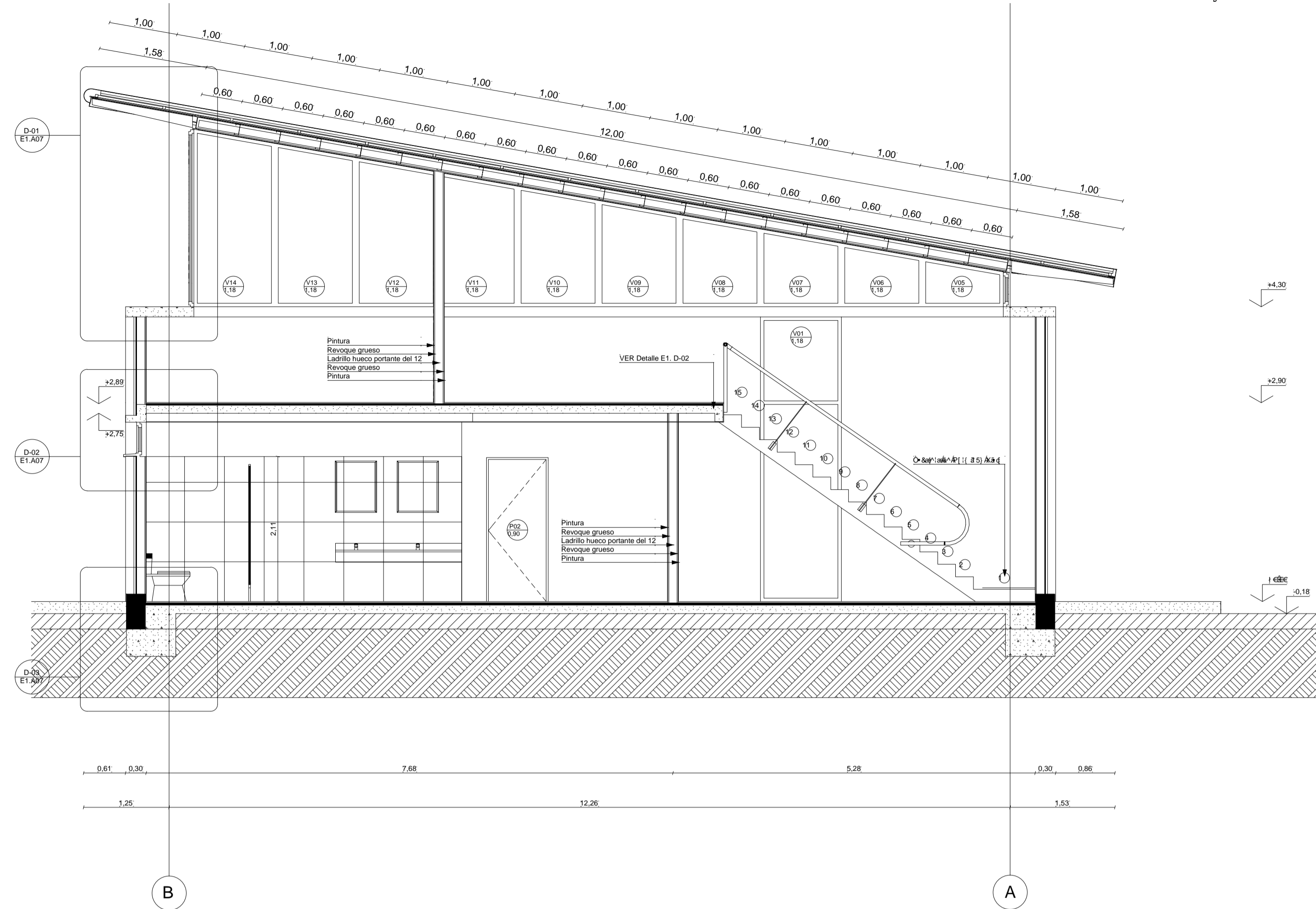
E1. Corte 1-1
