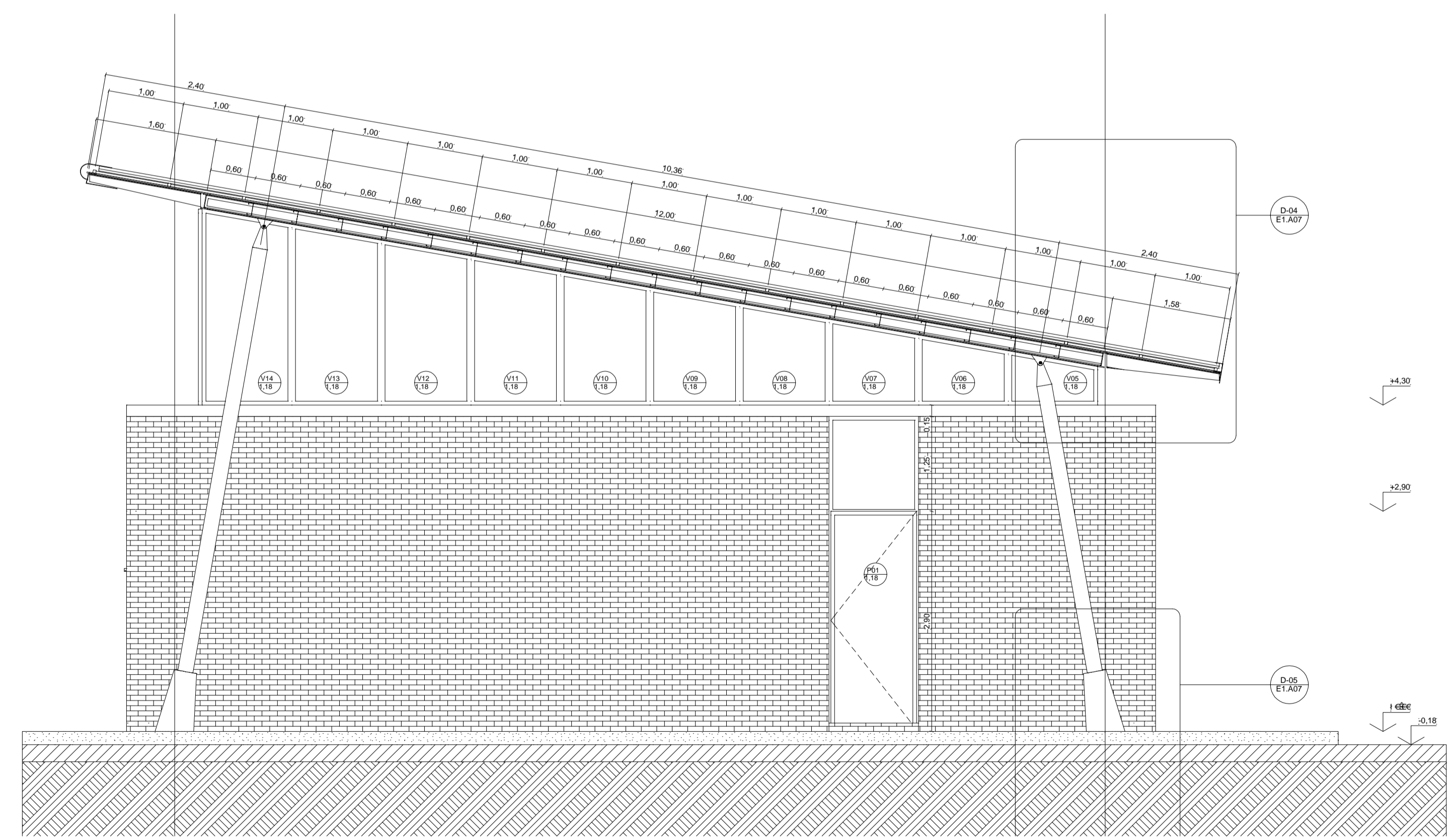
E1. Corte 2-2
