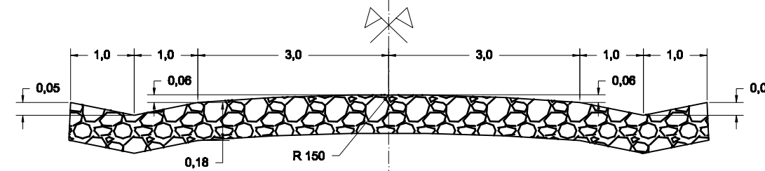
Perfil del corte A-B
