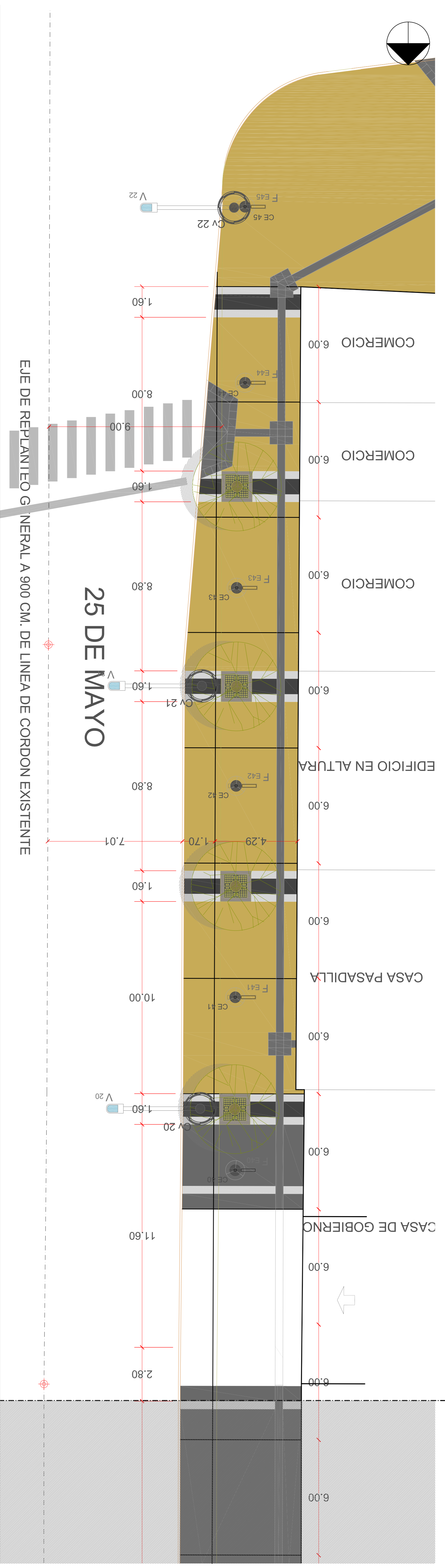
SECTOR SUR | CALLE 25 DE MAYO | JUNTAS DE DILATACION | 1 : 100
