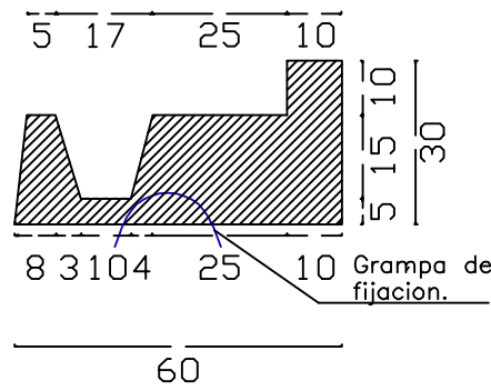
DETALLE A (marco)
