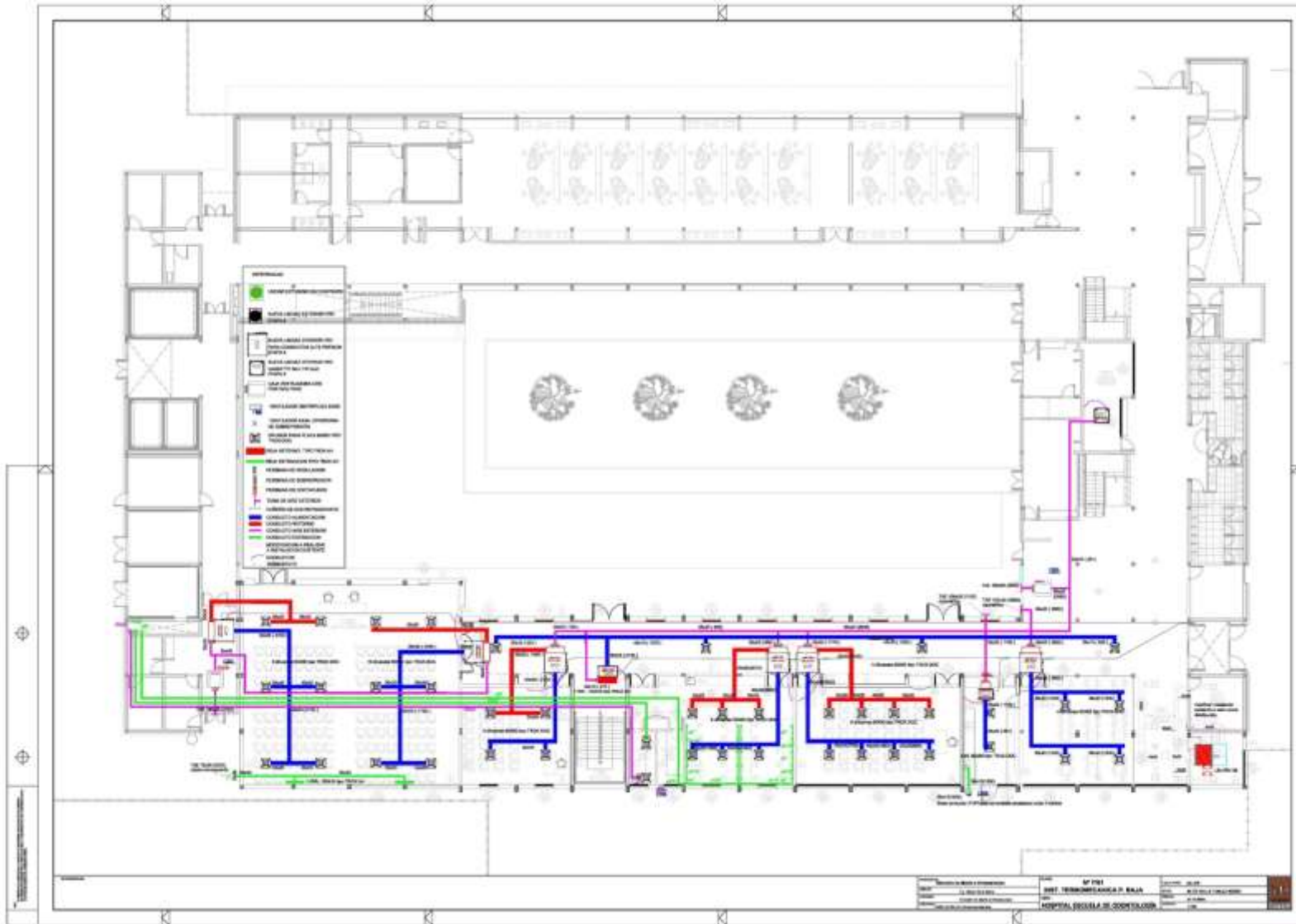
Figura N° 8: Esquema del sistema termomecánico en planta baja.
