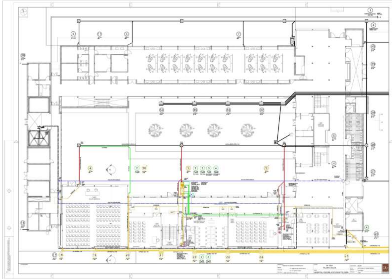
Figura N° 11: Esquema de instalaciones sanitarias de agua potable y cloacal.
