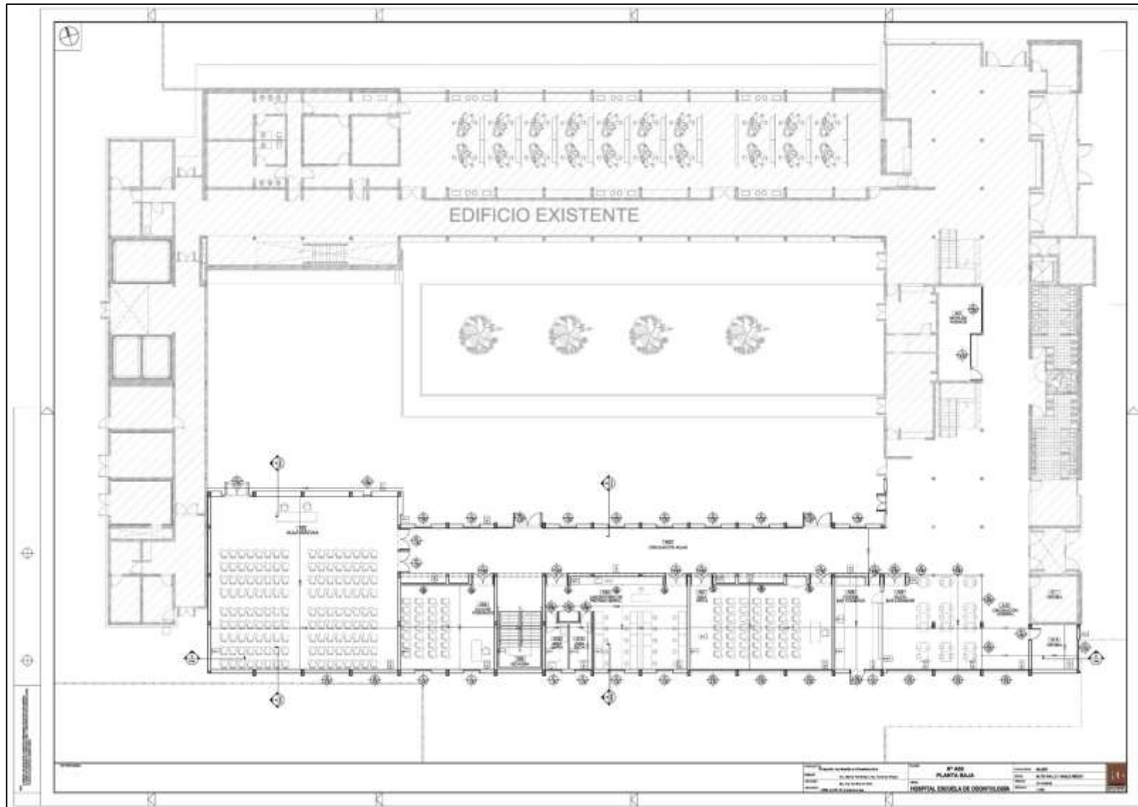
Figura N° 4: Plano de la planta baja – etapa 2.
