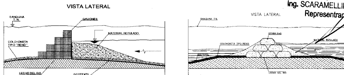
Figura N° 1: Croquis Vertederos Tipo para situación de aguas bajas
